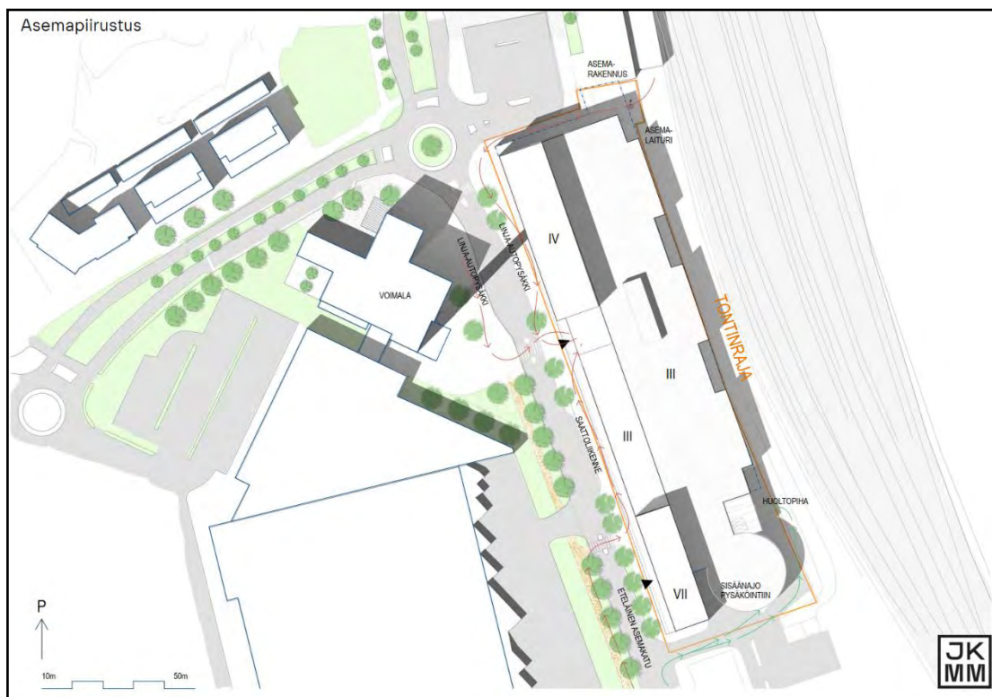
Kuva 1. Kohteen asemapiirros.
