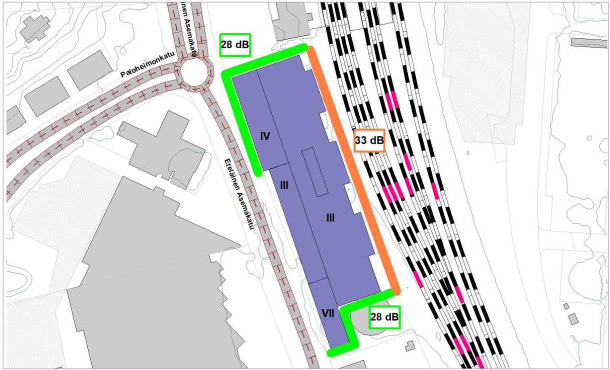
Kuva 18 Julkisivuille muodostuvat 28 dB ylittävät suositukset ulkovaipan äänitasoerovaatimuksiksi \Delta L_A , vaad (A-insinöörit Oy 2026).
