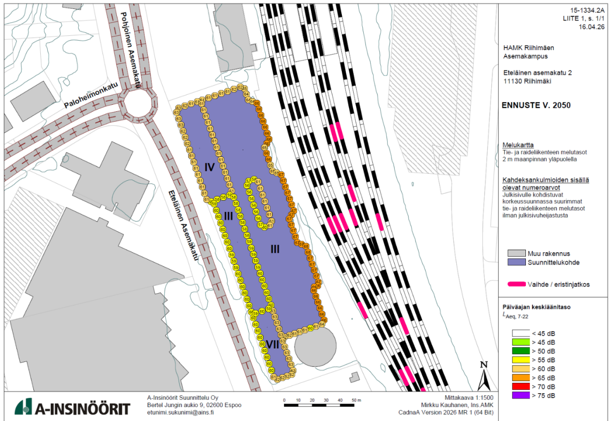
Kuva 17 Liikennemeluselvitys. Päiväajan keskiäänitaso ennustilanteessa vuonna 2050 (A-insinöörit Oy 2026).
