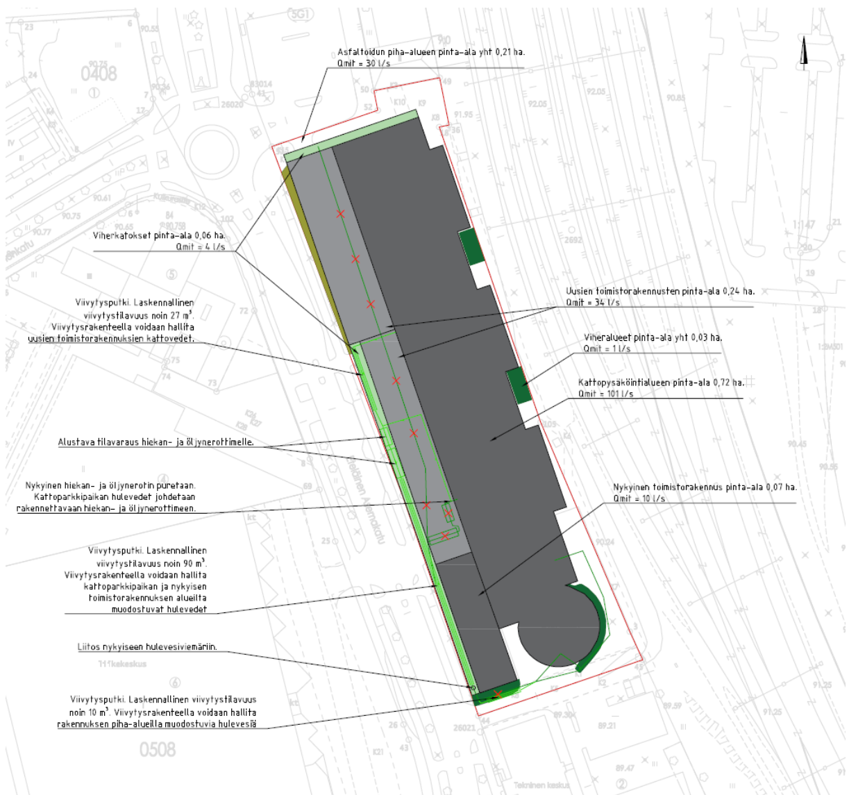
Kuva 20 Asemakaavamuutosalueen hulevesiselvityksen perusteella hulevesiä voidaan viivyttää kaavamuutosalueella 1 \text{ m}^3 / 100 \text{ m}^2 vettä läpäisemätöntä pinta-alaa kohden. Tarvittavat viivytysrakenteet sekä hiekan- ja öljynerottimet mahtuvat rakennusten ja Eteläisen asemakadun väliselle alueelle, ulokekatosten alle. Lähde: AFRY Finland Oy.
