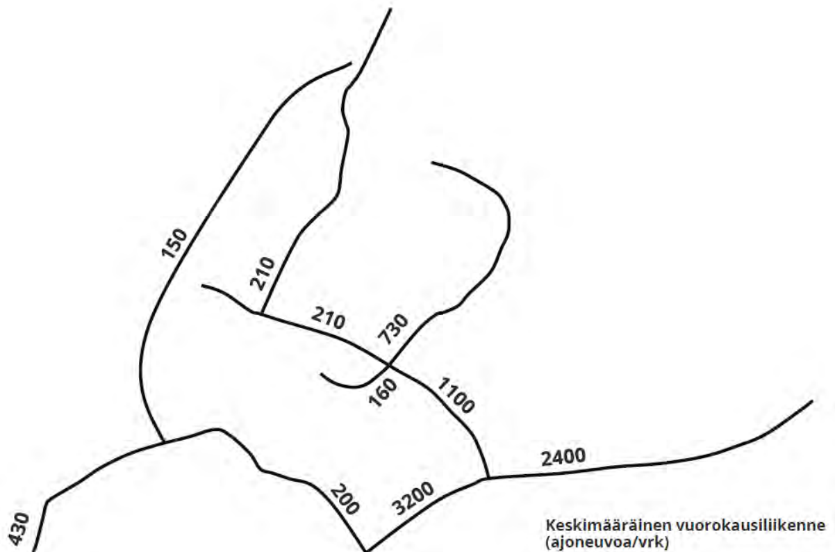
Kuva 21. Arviodut ajoneuvoliikennemäärät vuorokaudessa Kokonharjun asuinalueella ja sen lähiympäristössä. Kokonharjun liikenne-ennuste, Destia Oy.
