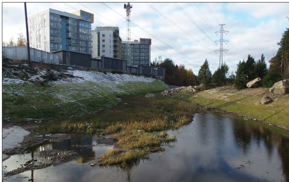
Kuva 17. Esimerkkikuva hulevesien viivytysaltaasta. Altaan reunoille on toteutettu eroosiosuojaus eroosiomatolla. Eroosiomatto nopeuttaa ruuhonsiementen kasvua sekä kasvuston kehitystä, mikä suojaa pintoja eroosiolta.
