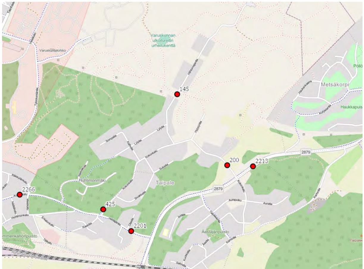
Kuva 6. Suunnittelualueutta ympäröivän liikenneverkon liikennemäärät (KVL) v. 2020–2022. Kuvan lähde: Riihimäen liikennetiedot Destia Smart View -palvelussa.
