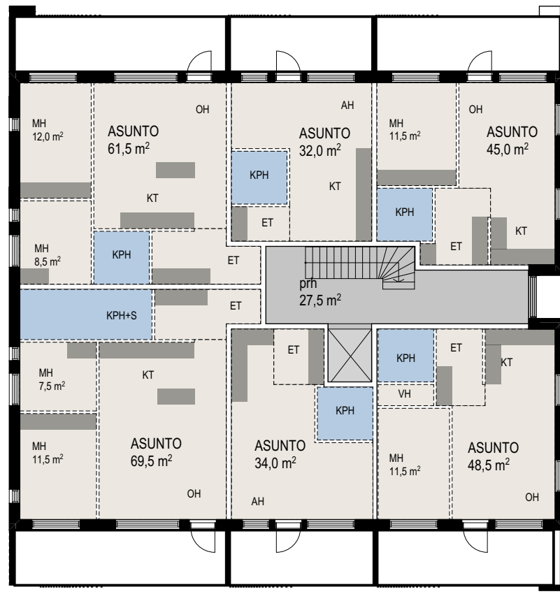
RAKENNUS 2 / 2.-4.kerros
