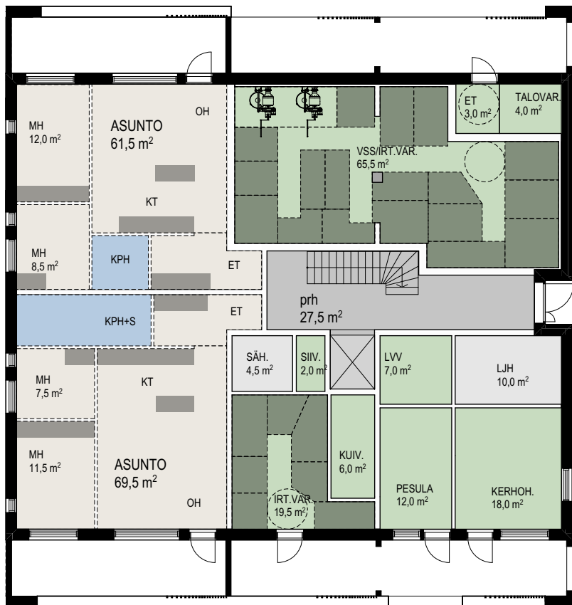
RAKENNUS 2 / 1.kerros
