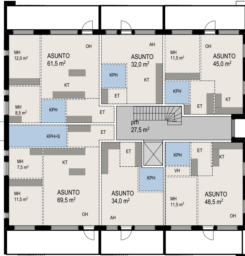
RAKENNUS 1 / 2.-4.kerros
