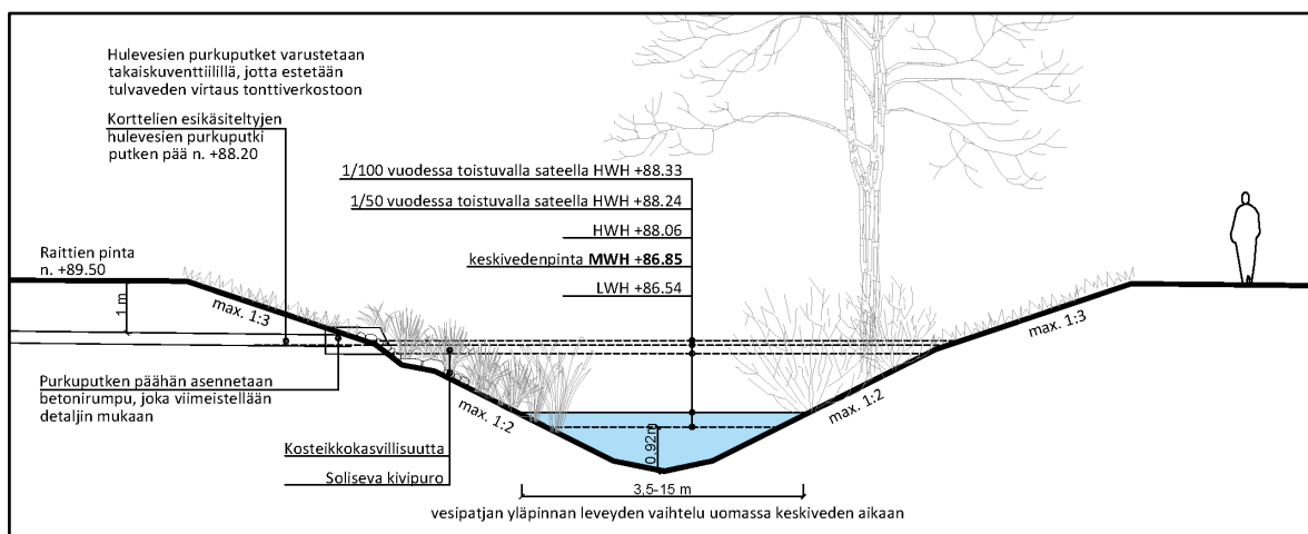
Kuva 8. Uoman periaateleikkaus ja korttelien hulevesien purkuputken pää betonirummulla. Ks. Liite 5.
