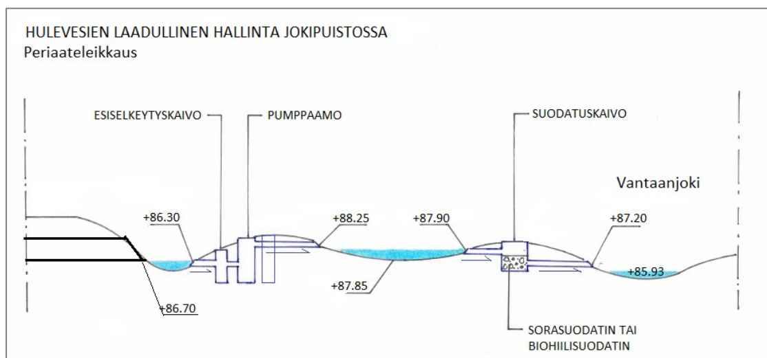
Kuva 10. Hulevesien laadullisen hallintarakenteen periaateleikkaus
