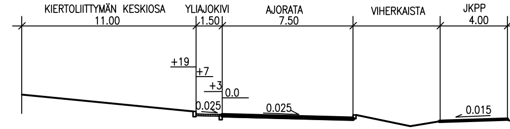
TYYPPIPOIKKILEIKKAUS 1:250
