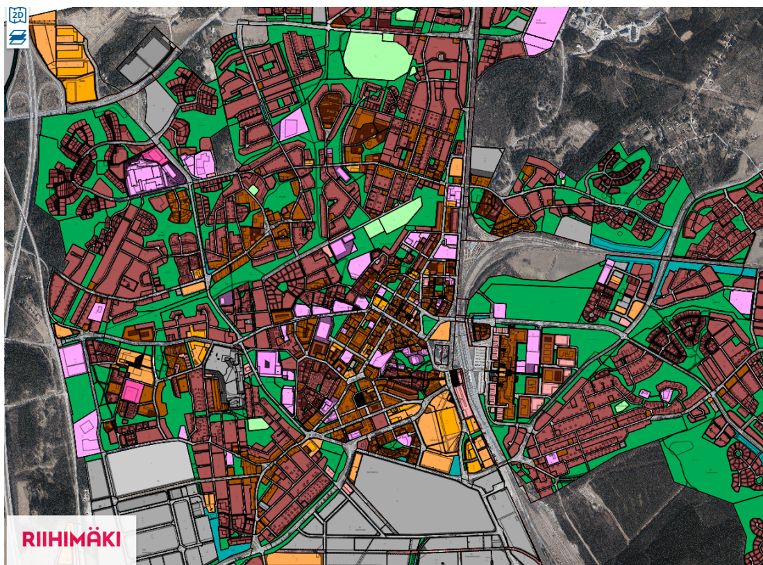
Kartta. Riihimäen keskustan ja asemanseudun alueen asemakaava.
