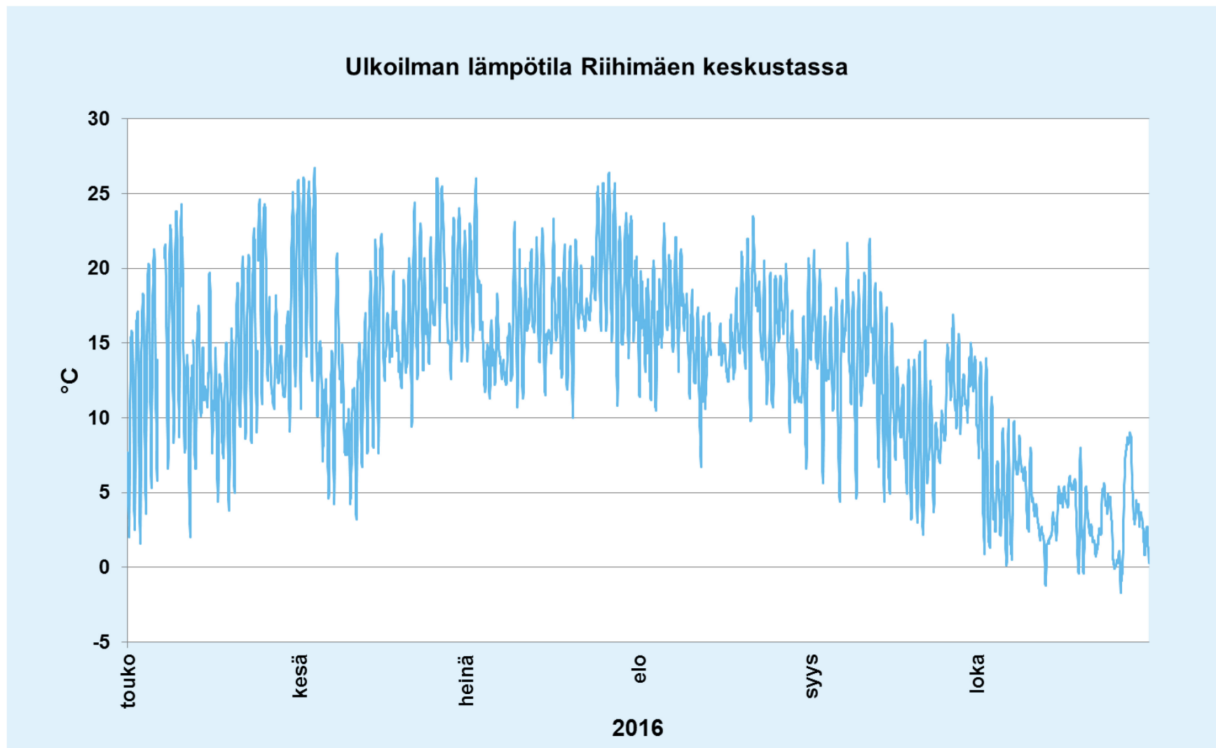
Liitekuva 1 Mittausjaksolla 1.5.–31.10.2016 havaittu ulkoilman lämpötila tuntiarvoina (°C) Riihimäen keskustassa Kolmiopuistossa.
